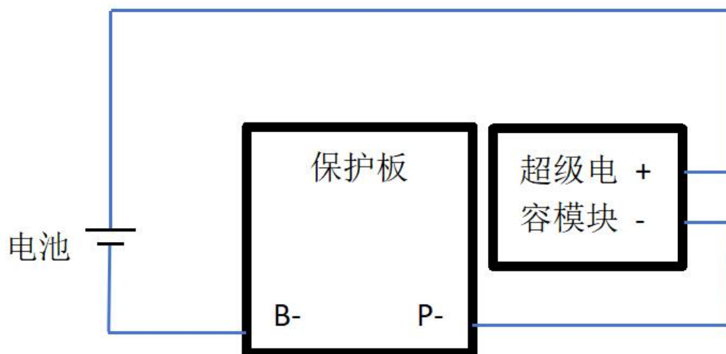
图 1 应用于带保护板的电池组
