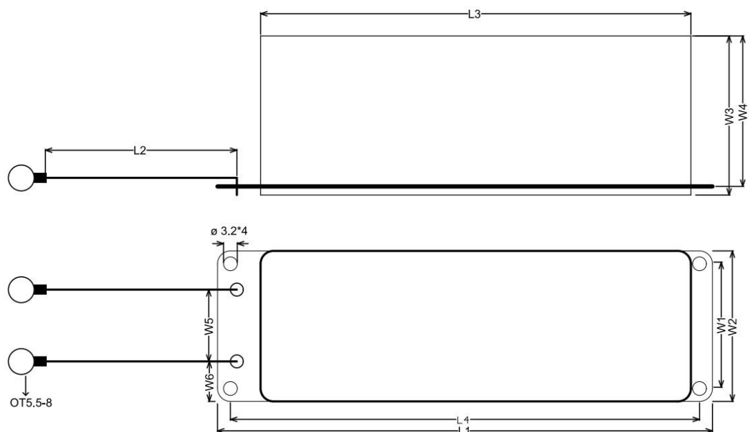
图 2 规格尺寸
