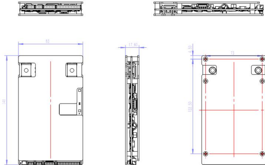
JK-BD4AxxS-6PRG 外形尺寸
