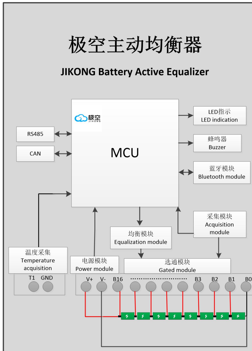
NY-B2A16S-TH 结构框图
