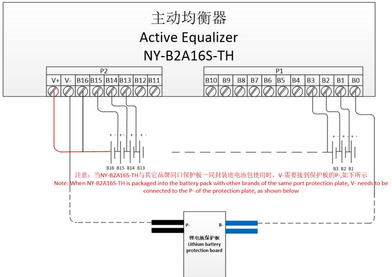
NY-B2A16S-TH 接线图
