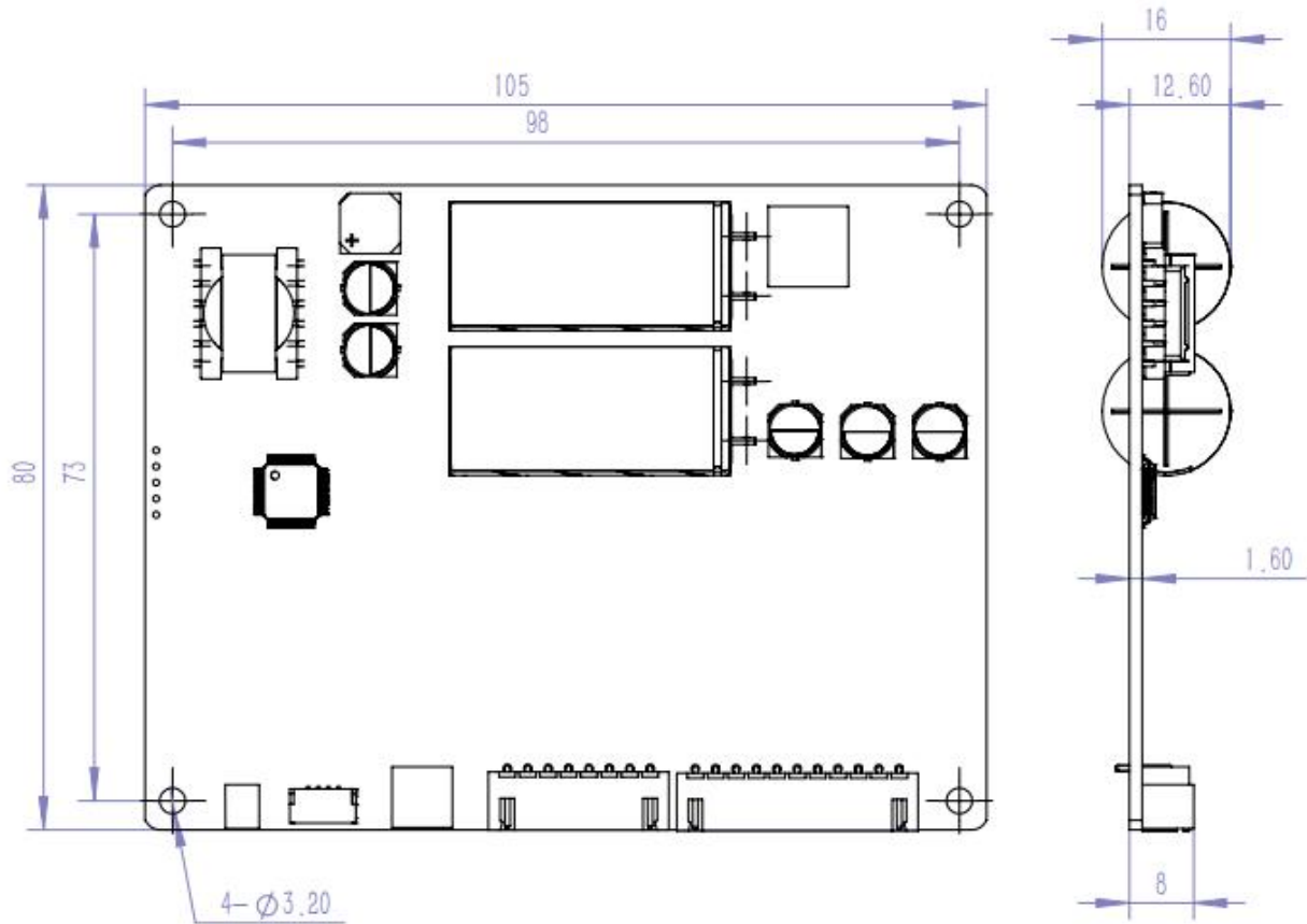
NY-B2A16S-TH 外形尺寸
