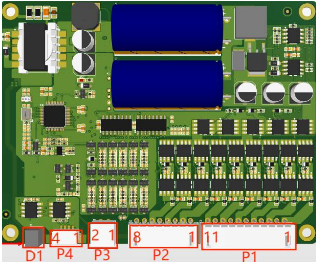
NY-B2A16S-TH 连接器示意图
